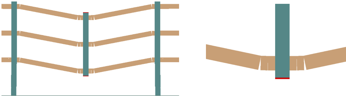
Figure (13) Numerical Crack Pattern [by ELS Software].
